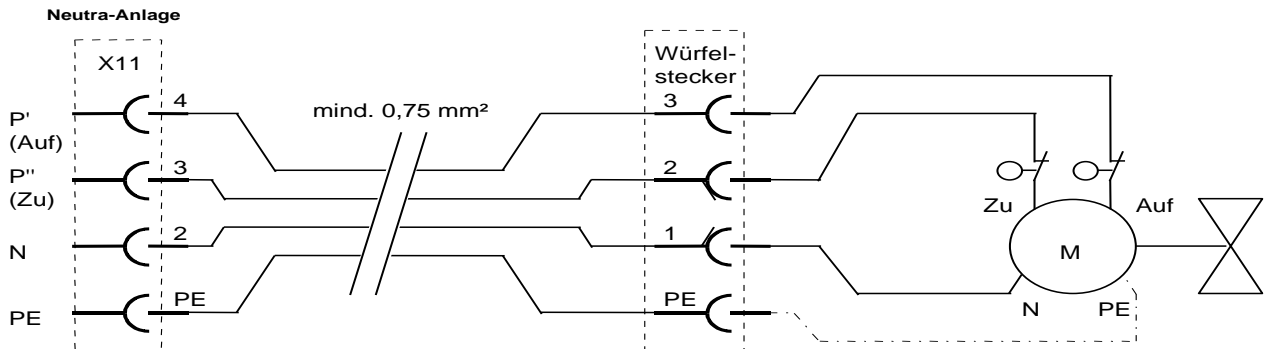
Bild 3.2: Anschluss Motorkugelhahn
