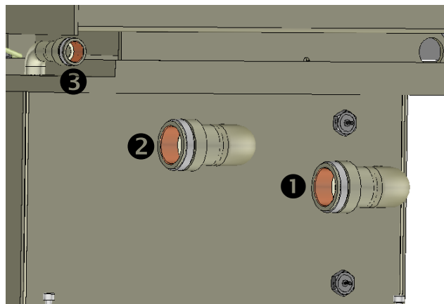
Bild 2.3: Sanitäranschlüsse
